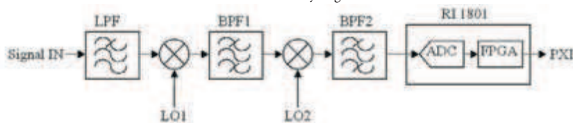
Fig 1. Förenklad arkitektur för spektrum- och I/Q modulations-analys. Frekvensen hos LO1 kan vara styrbar medan frekvensen hos LO2 kan vara fast.
